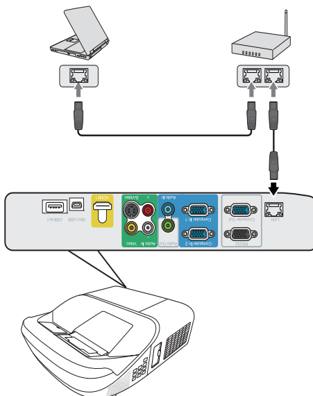
(Пример подключения)
