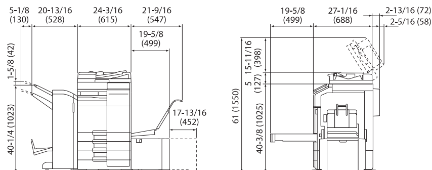
Основной блок + DF-632 + FS-536 SD + PC-216 + LU-302 + MK-730 + CU-102
