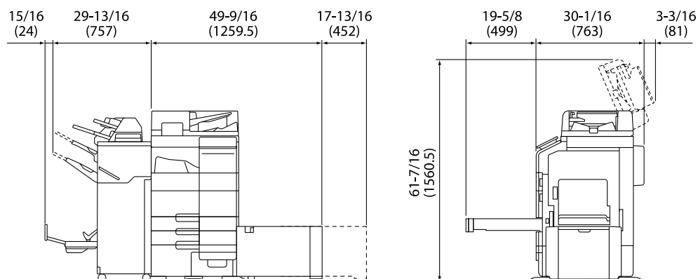
Основной блок + FS-540 SD + LU-205 + CU-102
