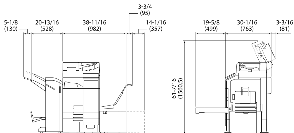
Основной блок + FS-539 SD + LU-303 + MK-730 + CU-102 Единица измерения: дюйм (мм)
