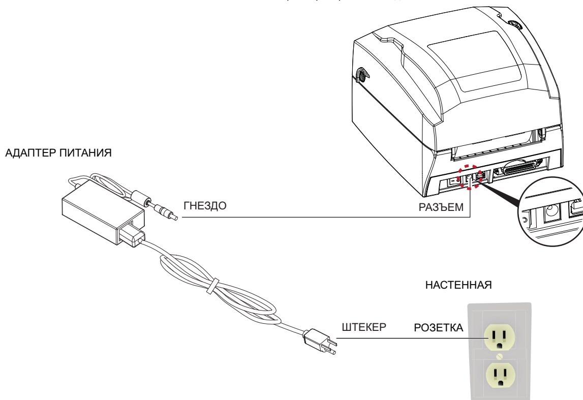
Принтер штриховых кодов G300
