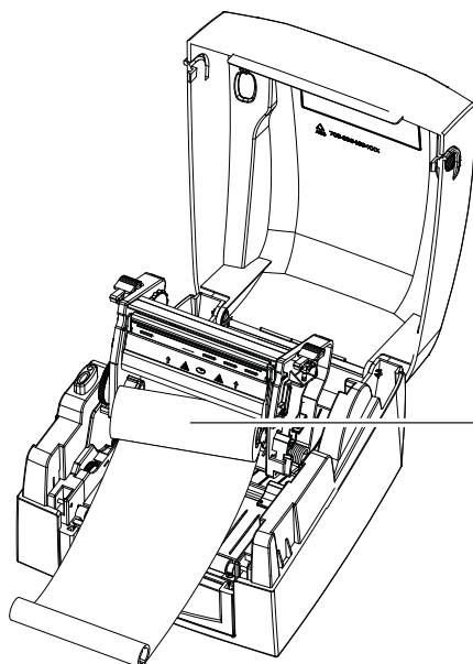
МОДУЛЬ ПОДАЧИ ЛЕНТЫ
