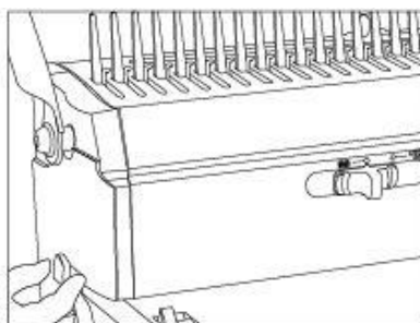
Рис.2 Выставьте регулятор глубины пробива в нужную позицию.
